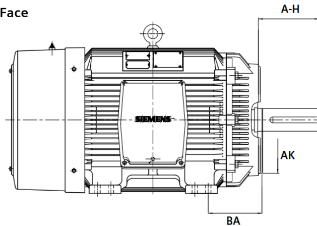
D-Flange
