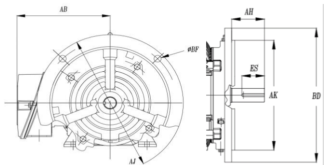
D-Flange
