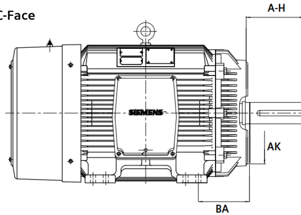
D-Flange
